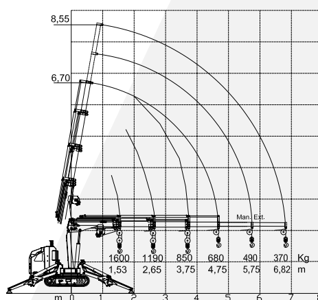
MCR30 Plus + Winch 800kg load chart
